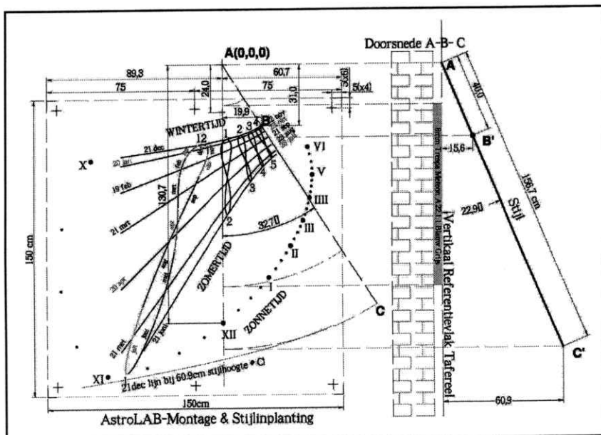
Fig. 5. De montage-instructies.
