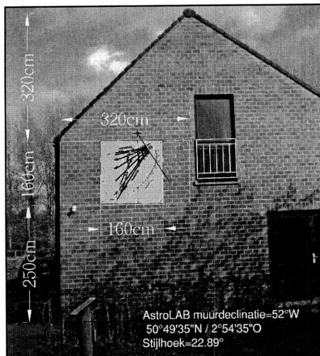
Fig. 1. Een kijkje op de westelijke muur van het AstroLAB I met aanduiding van de voorziene plaatsing van de zonnewijzer.
