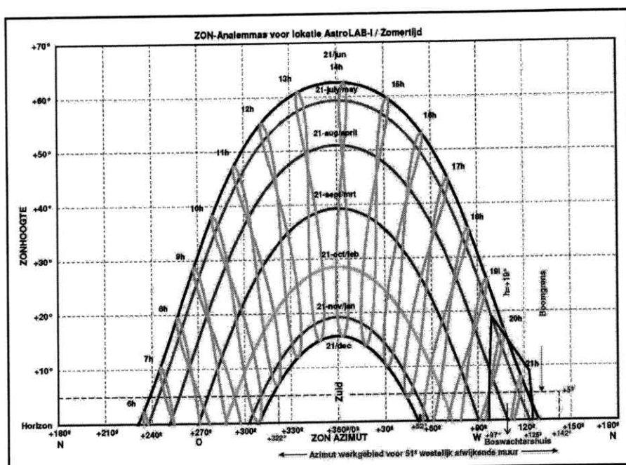
Fig. 3. Zonnetraject met boomgrens, boswachterhuis en schaduwgrens.
