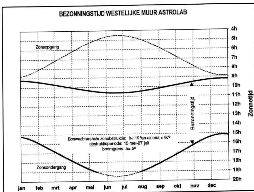
Fig. 2. Bezonningsstijlgrafiek.
