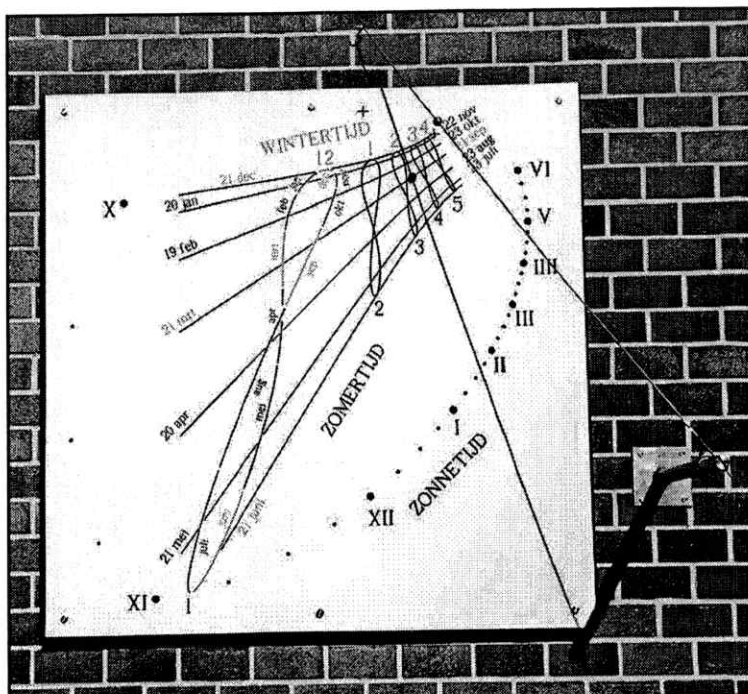
Fig. 7. De zonnwijzer van het AstroLAB I in Zillebeke. (Foto Franky Dubois)
